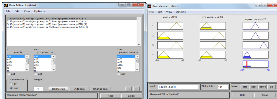
Рис. 3. Окно редактора RuleEditor
