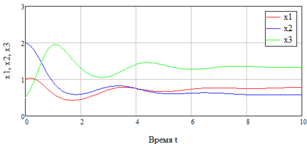
Рис. 1. График траекторий решений модели (1) при начальном условии x_1, x_2, x_3 = 1, 2, 0.5
