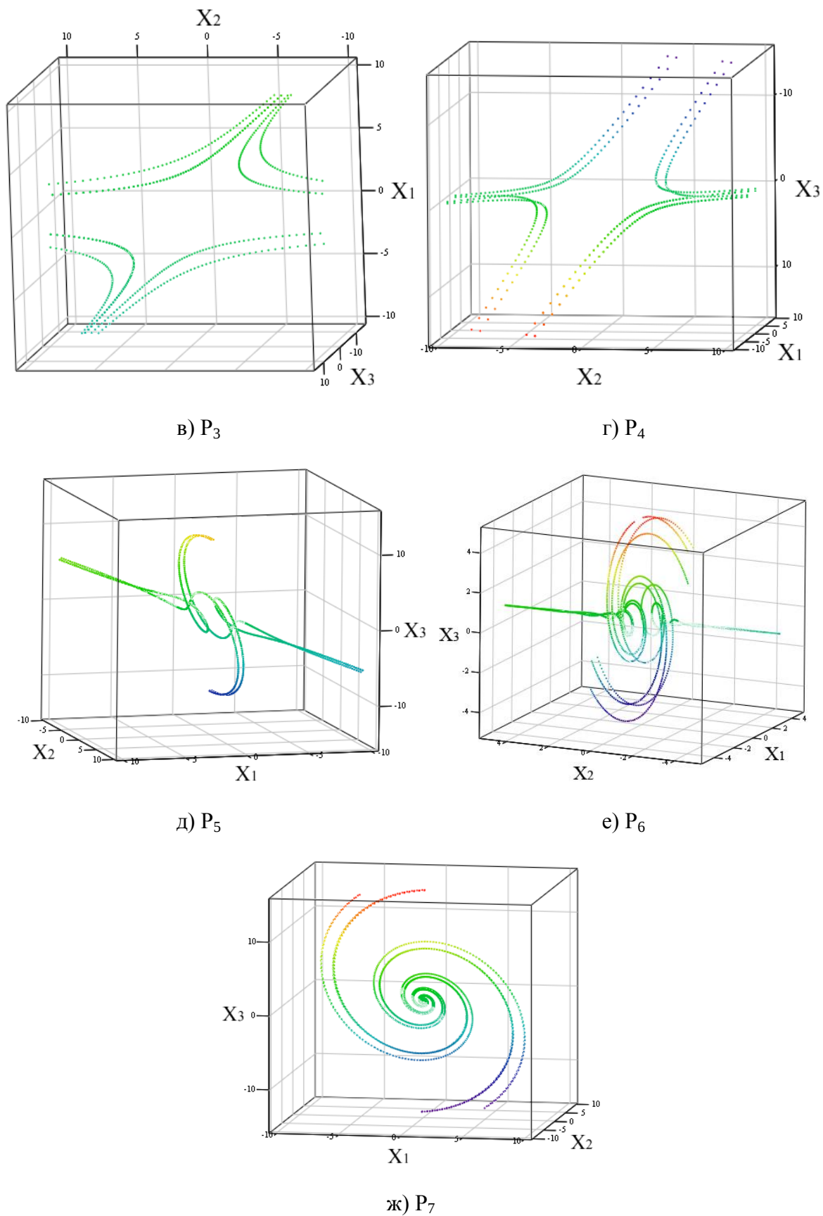
Рис. 2. Фазовые портреты в окрестностях стационарных состояний P_1 - P_7 модели (1)
